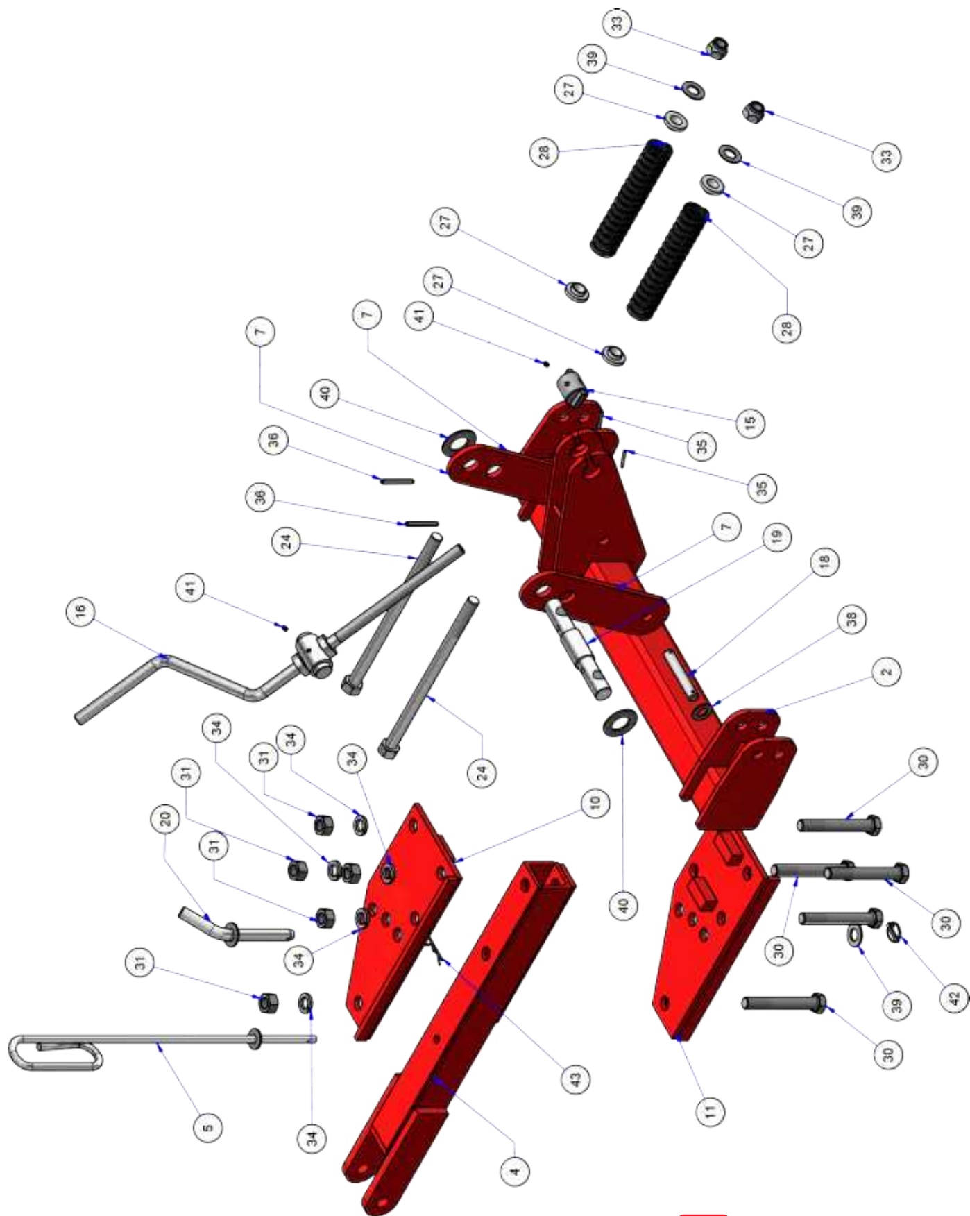
CONJUNTO TIRO TIPO A
